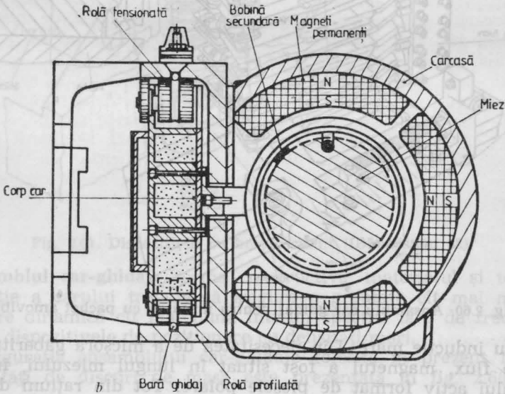
Fig. 2.58. Motor linear cu „bobină scurtă” pentru unități cu discuri încasetate (Infomag 44): a — dispozitivul de poziționare; b — secțiune transversală.
