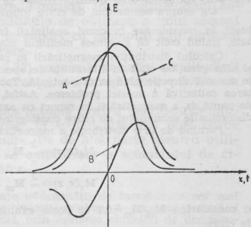
Fig. 2.20. Semnal de citire; ipoteza „arctangentă“ (după [2]):
