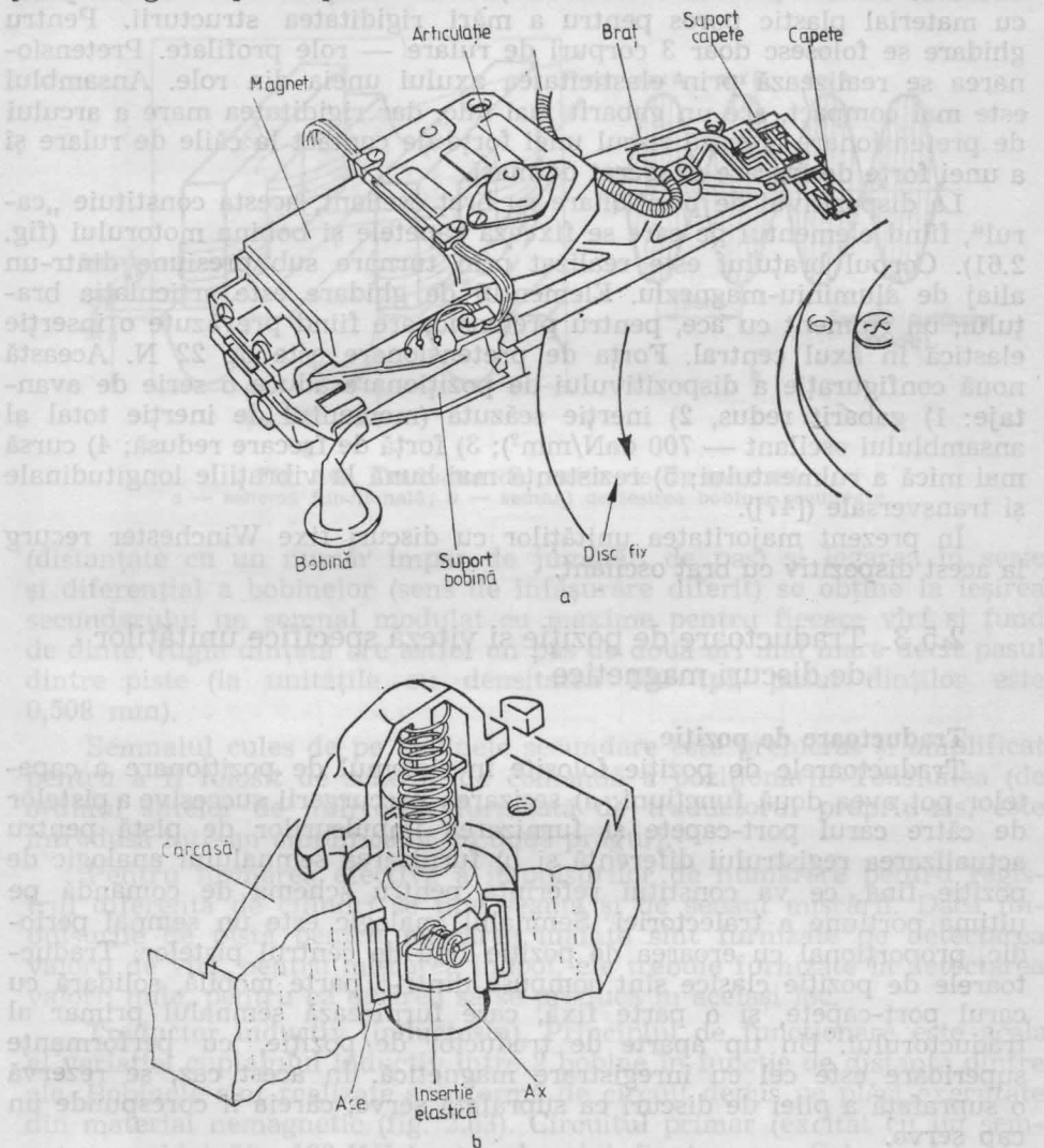
Fig. 2.61. Dispozitivul cu braț oscilant (IBM sistem 32).
