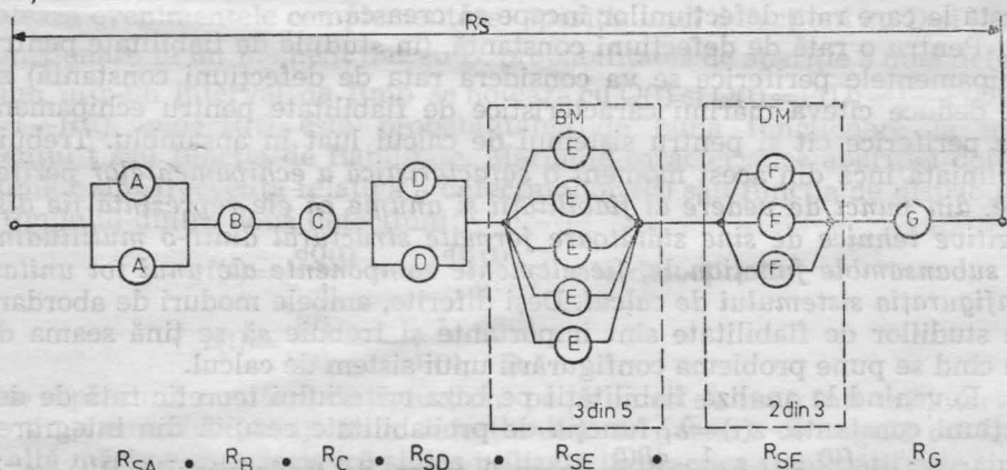
Fig. 1.10. Exemplu de schemã de fiabilitate pentru un sistem de calcul.
