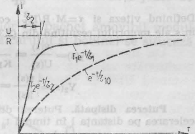
Fig. 2.54. Constanta de timp electrică a bobinei.
