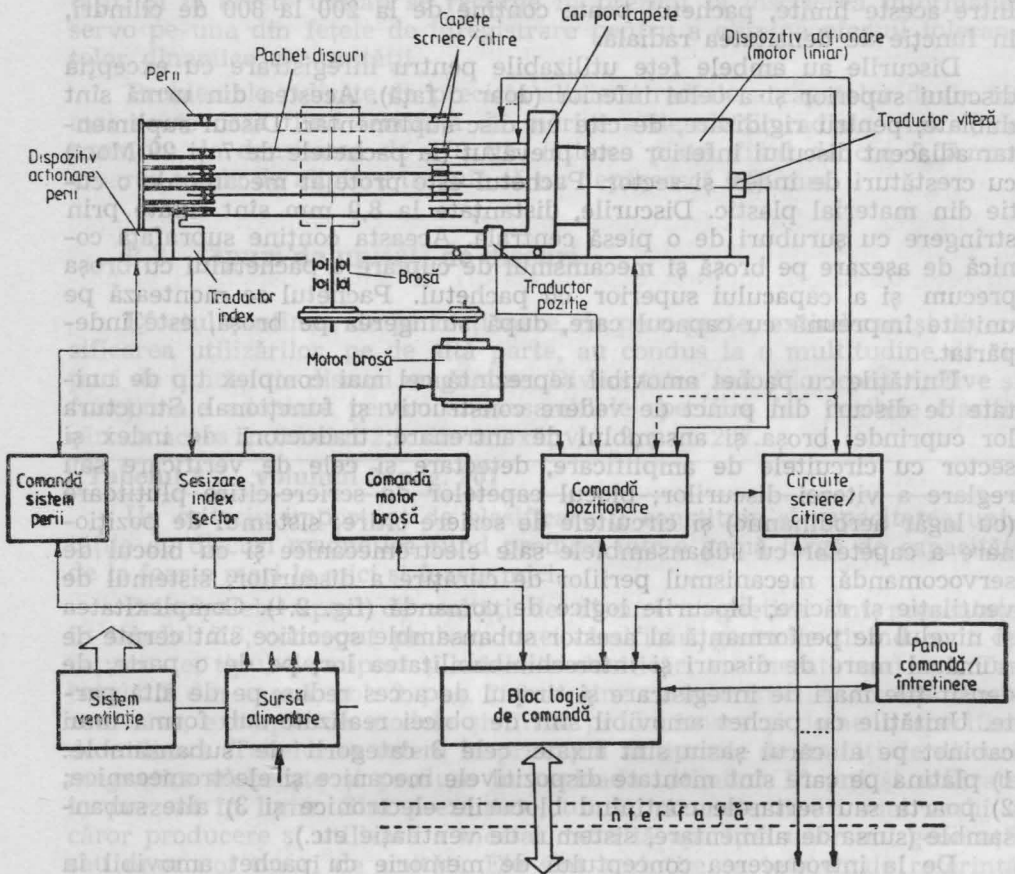
Fig. 2.4. Unitate de discuri cu pachet amovibil:
