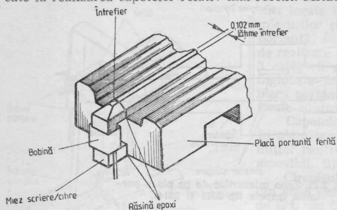
Fig. 2.27. Fixarea miezului de scriere/citire pe spatele plăcii portante la capul Winchester.
