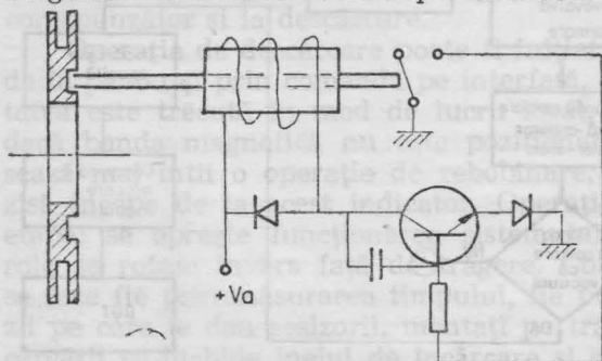
Fig. 3.45. Traductor de protecție fișier cu rețineri electromagnetice.
