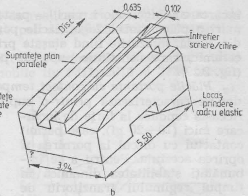
Fig. 2.38. Plăci portante cu contact temporar:
