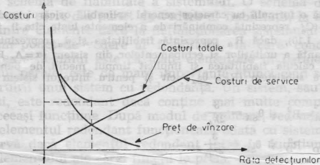
Fig. 1.11. Diagramă estimativă costuri funcție de rata defecțiunilor.
