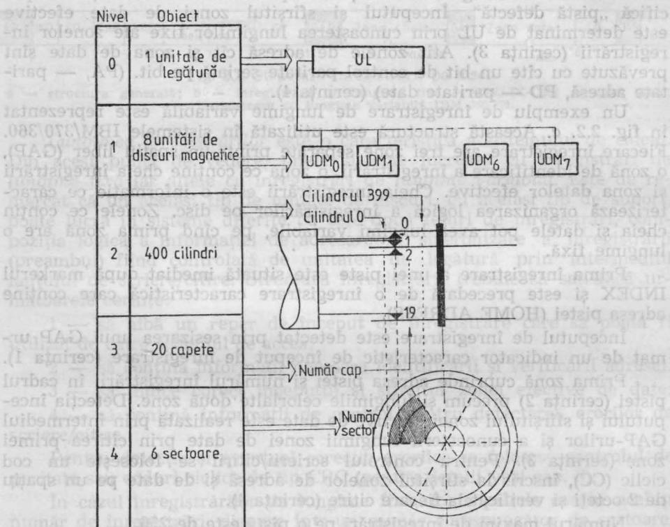
Fig. 2.3. Nivele de adresare la un subsistem de 8 unități de discuri.
