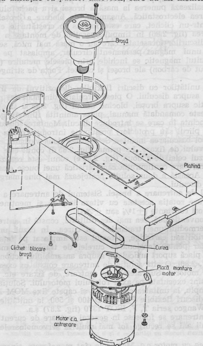
Fig. 2.86. Broșa și sistemul de antrenare cu motor c.a. la unitate cu pachet amovibil tip m 3330 (Memorex 3670).
