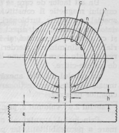
Fig. 2.18. Schema funcțională a capului de înregistrare.
