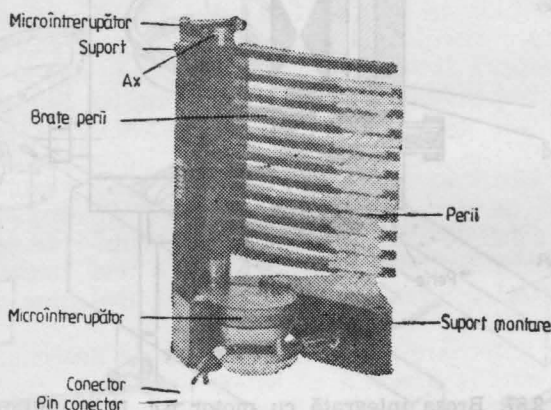
Fig. 2.88. Ansamblul periiilor de curățire (unitate BASF 6114).
