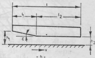
Fig. 2.31. Tipuri de lagăre utilizate în construcția capetelor de scriere/citire: a - lenticular; b - teșit.
