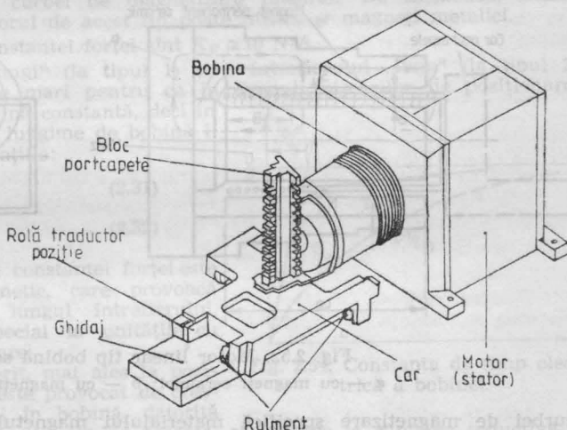
Fig. 2.50. Dispozitiv de poziționare cu motor linear (CDC BR1A1).
