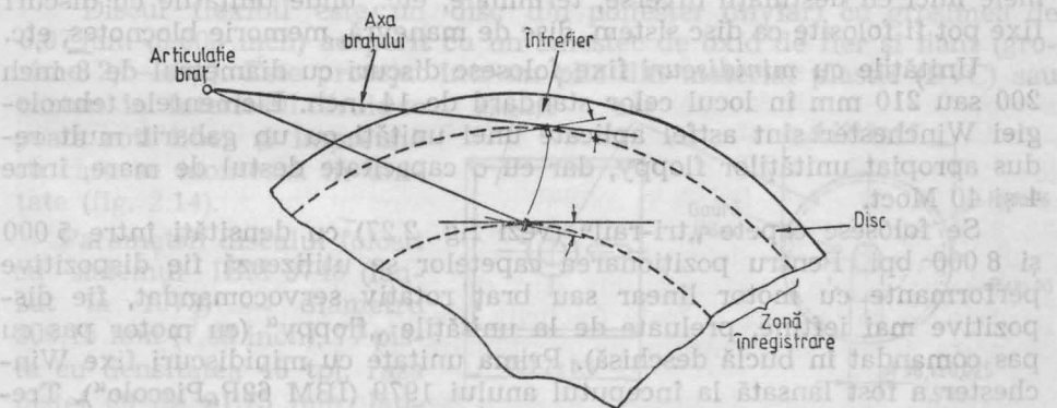
Fig. 2.12. Geometria sistemului de poziționare cu braț oscilant.
