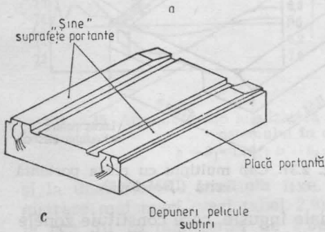
Fig. 2.38. Plăci portante cu contact temporar:
