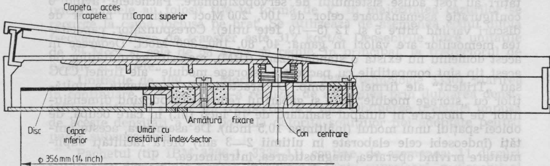
Fig. 2.8. Caseta „cartridge“ cu montare frontală (tip IBM 2315) după standard ISO/TC97/SC10/109.
