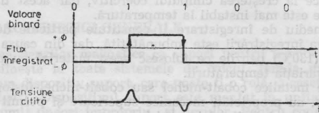
Fig. 3.1. Metoda de înregistrare NRZI.
