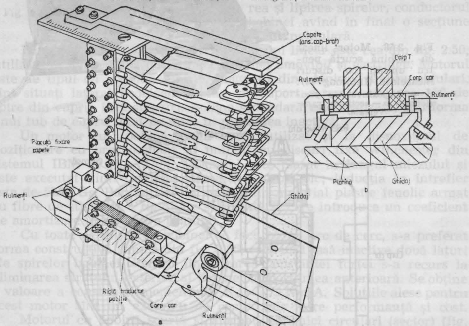
Fig. 2.60. Ansamblu car-ghidaj pentru unitățile cu pachet amovibil.
