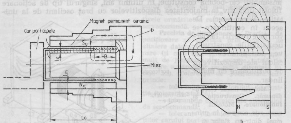
Fig. 2.52. Motor linear tip bobină scurtă:
