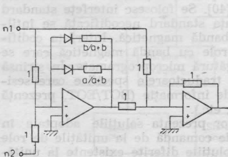
Fig. 3.34. Schemă de realizare a funcției de eroare.
