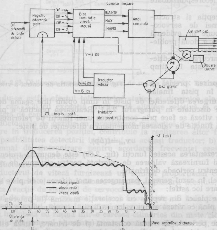
Fig. 2.70. Principiul schemei de servocomandă la unitatea (CDC9645).
